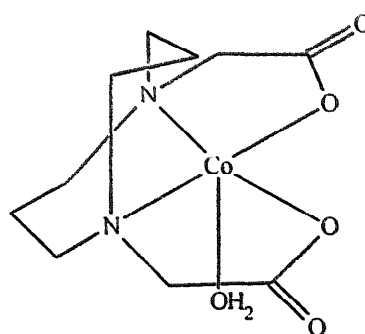
[Co(dacoda)H 2 O]
